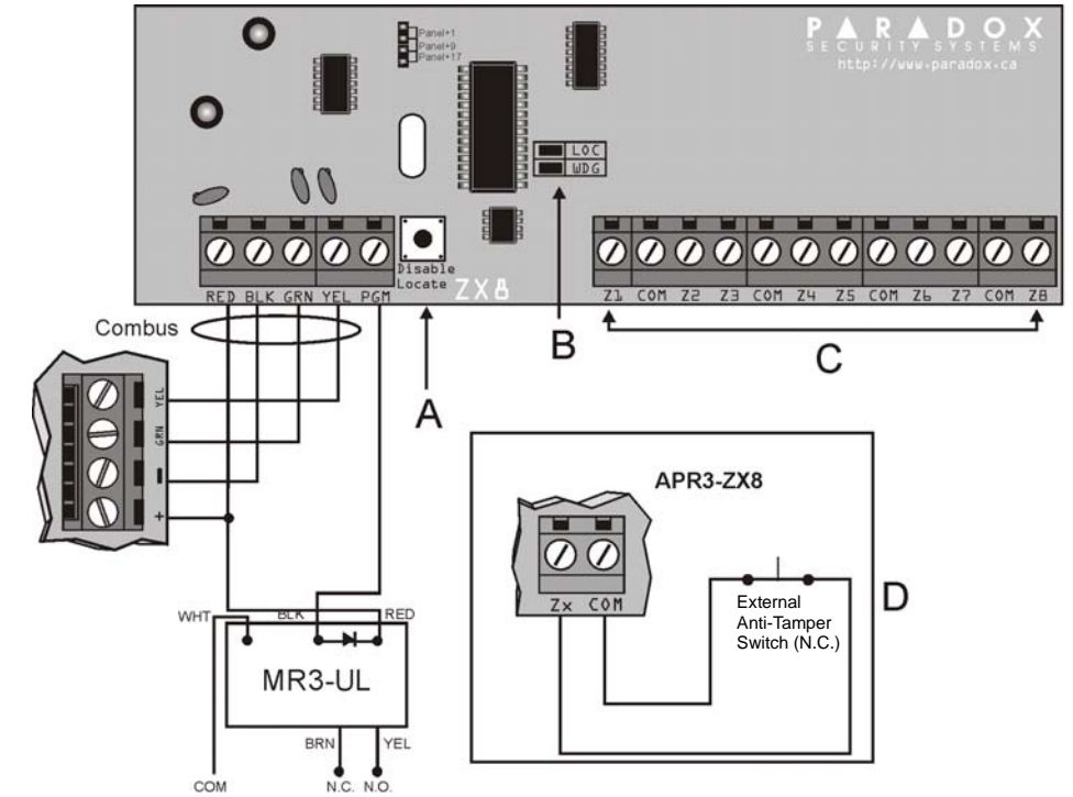
Figure / Figura 1: ZX8 Connection/Conexión/Connexion
